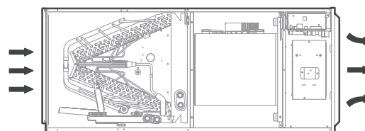
Horizontal droit
