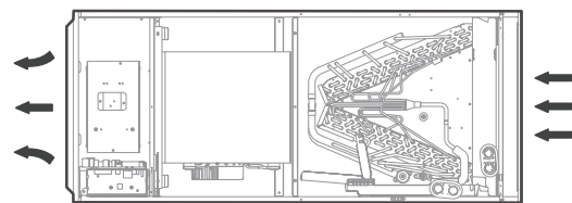
Horizontal left
