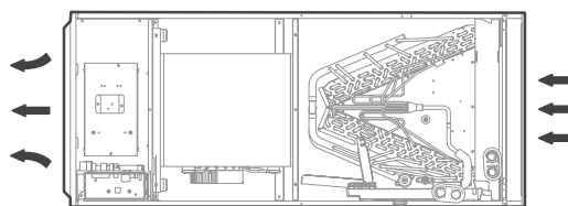
Horizontal gauche
